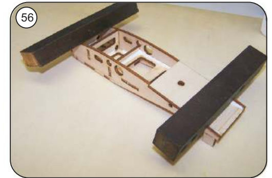
Verstärkungsauflage M 7 einkleben und gesamte Einheit bis zum Durchtrocknen mit Gewichten auf das Baubrett pressen
