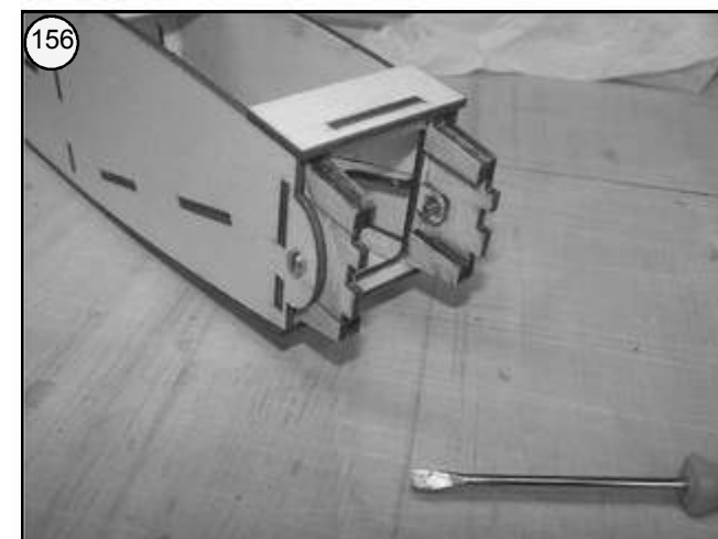
Bild 156 - Baugruppen in den Rumpfkopf einschrauben.
