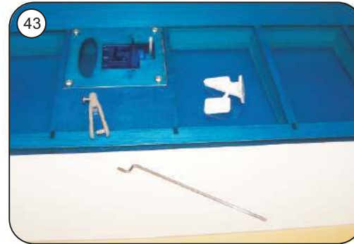
Anlenkungsgestänge aus den Teilen F 37, F 38 und F 39 vormontieren
