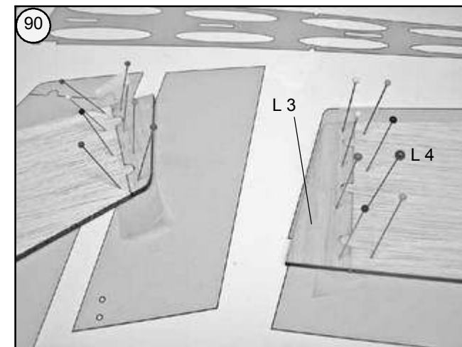
Bilder 89 und 90 - Randbogen L 3 an das Seitenleitwerk L 4 kleben und fixieren.
