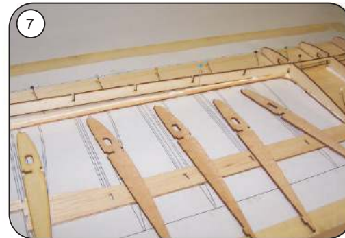
Kammholm F 10 aufleimen und Rippen F 11 bis F 16 nach Plan vorsortieren
