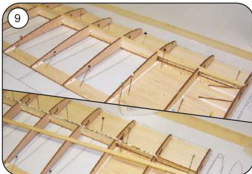
Oberen Hauptholm F 17 aufleimen, auf gute Verklebung achten !
