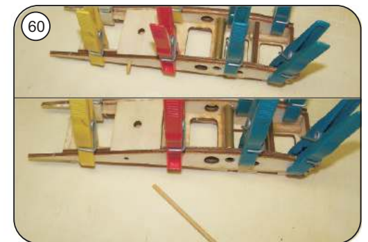
Klebestellen bis zum Aushärten mit Klammern fixieren, Buchendübel sofort entfernen
