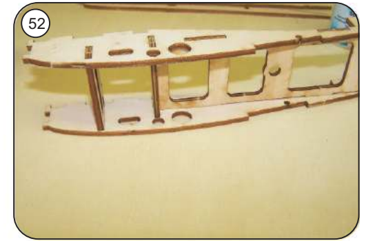
Gegenrippe M 1 aufstecken und anheften
