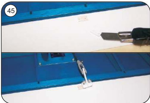
Bespannung im Auflagebereich des Ruderhorns entfernen, Befestigungsschrauben leicht eindrehen
