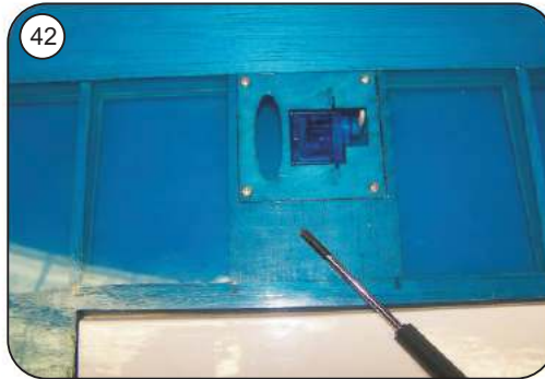
Servoeinheit in die Fläche einsetzen und mit den Schrauben F 36 verschrauben, Funktionsprobe durchführen
