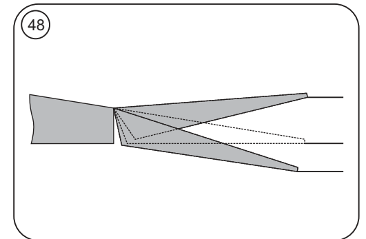
Ruderausschläge und Differenzierung gem. Skizze mit der RC-Anlage einstellen
