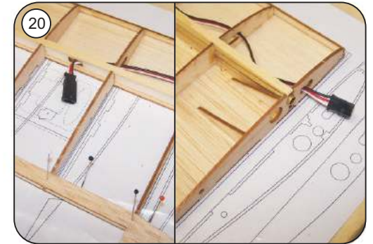
Servo- Verlängerungskabe einziehen
