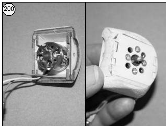
Bild 200 - Motor von der Innenseite durch den Motorspant der Motorhaube durchstecken und verschrauben.
