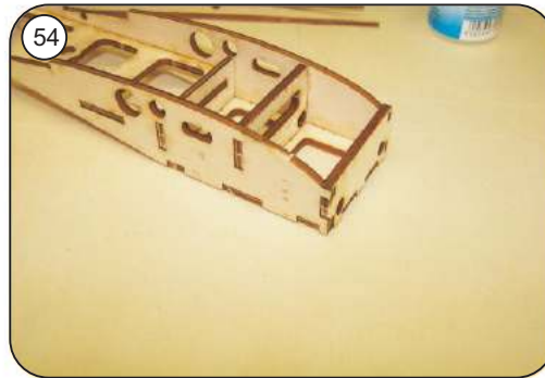
Spant M 6 einsetzen und anheften
