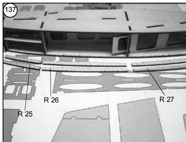
Bilder 137 und 138 - Je einen Rumpfgurt R 25 - R 27 innen zwischen den Spanten einpassen und einkleben.
