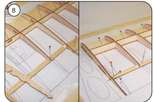
Rippen F 11 bis F 16 einleimen, Beplankungsteile dabei auf dem Baubrett aufnadeln
