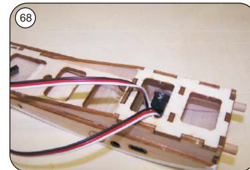
Buchsen aussen bündig einstecken und von der Innenseite mit Epoxy festkleben
