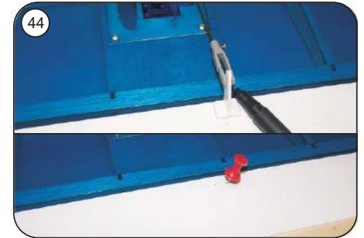
Gestänge am Servo einhängen, Ruderhorn-Position anzeichnen und in das Querruder einstechen
