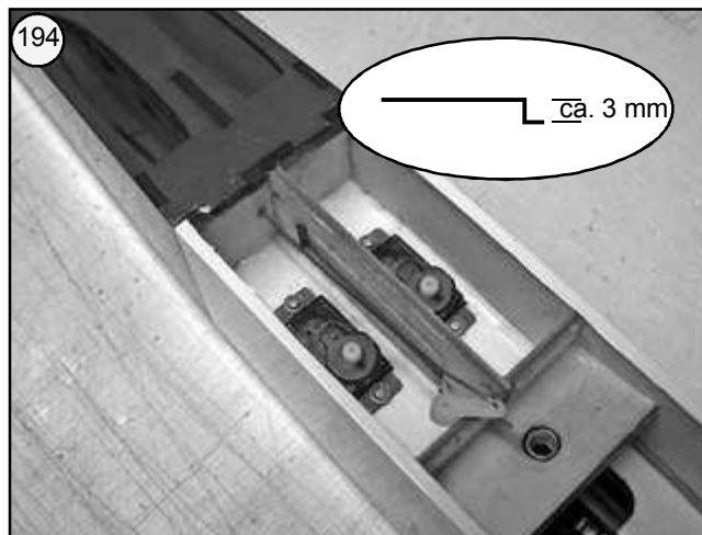
Bild 194 - Z - Gestänge nach Skizze biegen und in den Servohebel einfädeln. Gestänge in das Führungsrohr einschieben.
