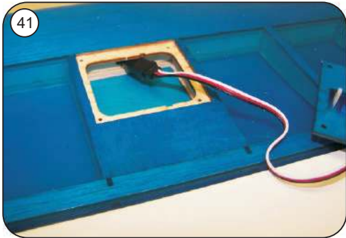
Servo mit dem Verlängerungskabel verbinden, evtl. mit Klebeband sichern
