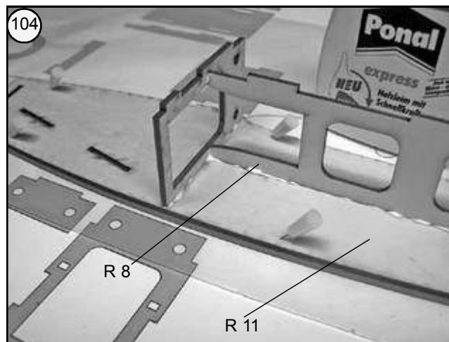
Bild 104 - Fertigen Innenrahmen auf die rechte Rumpfschienenwand R 11 kleben.
