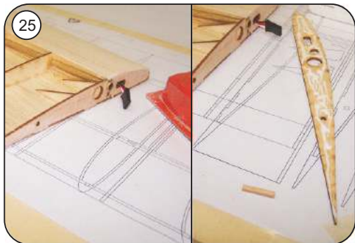
Überstände im Bereich von Rippe F 9 bündig verschleifen, Wurzelrippe F 27 satt mit Holzleim einstreichen
