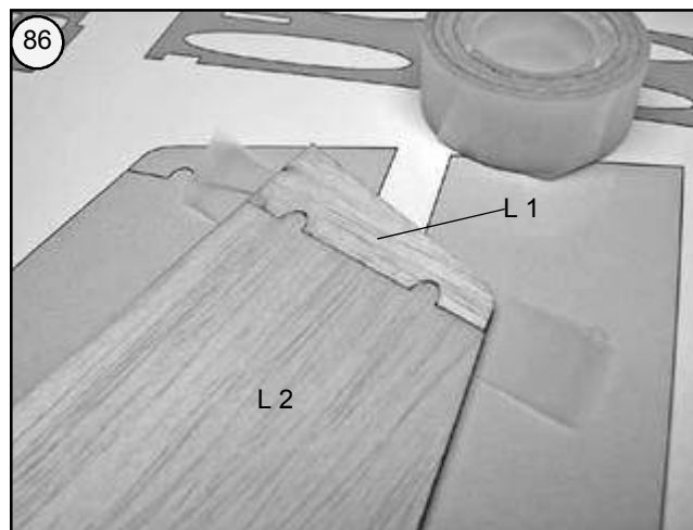
Bild 86 - Randbogen L 1 mit Tesafilm am Höhenleitwerk L 2 fixieren.
