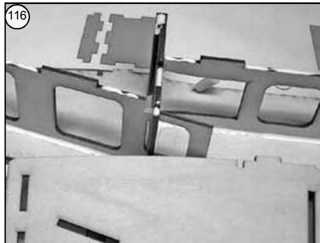
Bilder 116 und 117 - Die linke Rumpfseitenwand R 11 aufkleben. Auf korrekten Sitz zur rechten Seitenwand achten.
