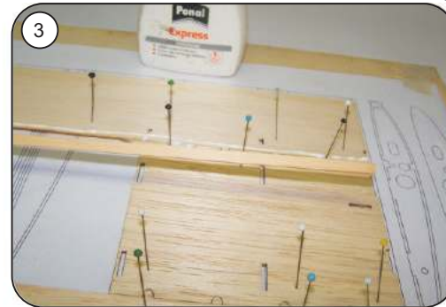
Hauptholm F 4 auf untere Nasenbeplankg. F 1 exakt nach Plan aufleimen
