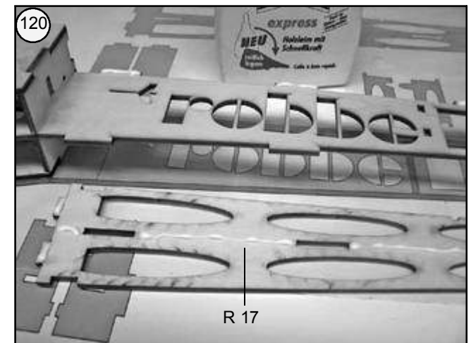
Bilder 120 und 121 - Den hinteren Rumpfdeckel R 17 auf den Leitwerksträger kleben.
