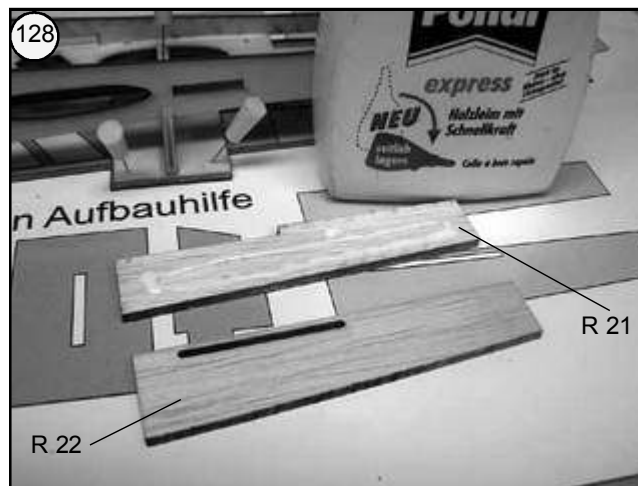
Bilder 128 und 129 - Den linken Rumpfabschluss aus den Balsateilen R 21 und R 22 deckungsgleich zusammenkleben.
