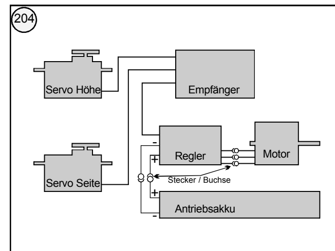
Bild 204 - Anschluss-Schema der RC- und Antriebskomponenten.
