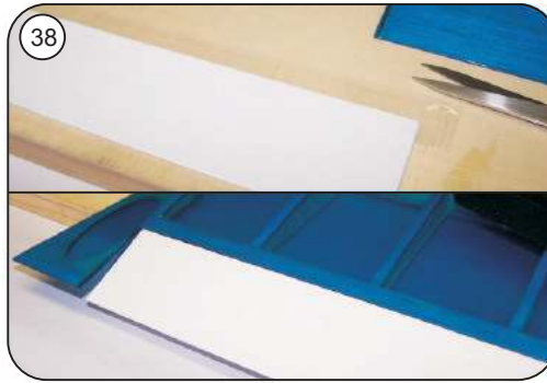
Zuerst die Oberseite ankleben, auf ausreichend Ausschlag nach unten achten
