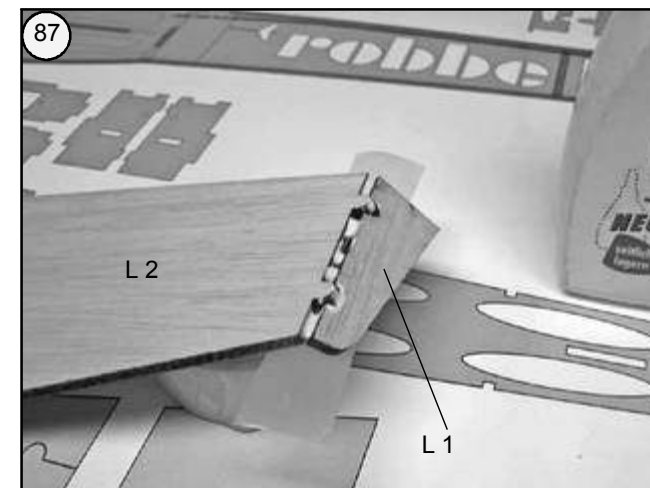
Bild 87 - Klebestelle mit Leim versehen.
