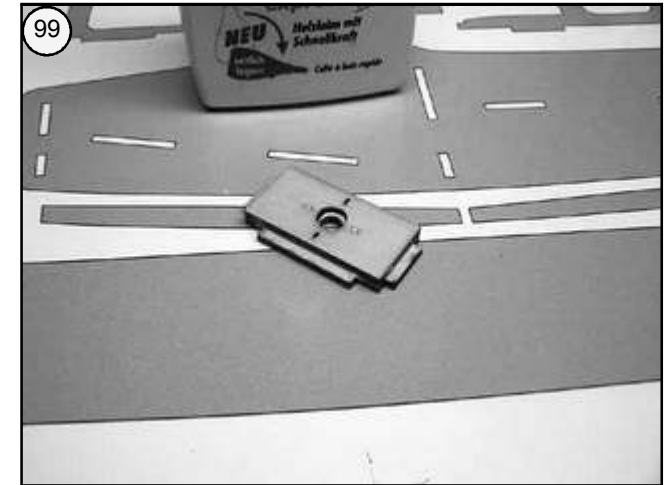
Bild 99 - Auf deckungsgleiche Bohrungen und bündig verlaufende Kanten achten.
