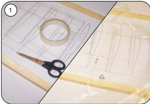
Bauplan auf das Baubrett aufkleben und mit PE-Folie abdecken
