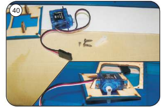
Servo mit RC-Anlage in Nullstellung bringen, langen Ruderhebel anschrauben, Servo in die Halterung schrauben
