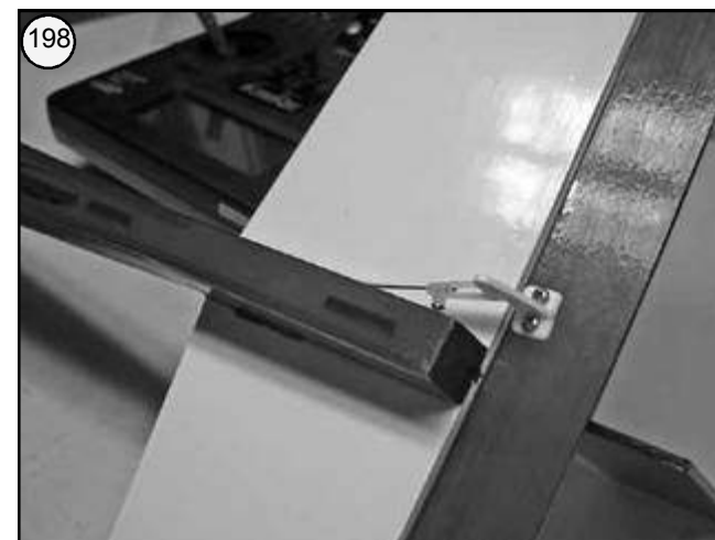
Bild 198 - Höhenruder in der gleichen Weise anlenken.
