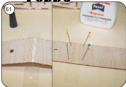
Obere Beplankung aus M 11 und M 12 herstellen
