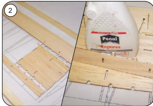
Untere Beplankungsteile F 1, F 2 und F 3 auf dem Plan ausrichten und verkleben
