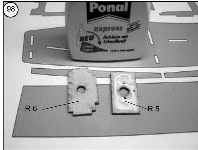
Bild 98 - Die Aufdopplung R 5 auf die Flächenhalterung R 6 kleben.
