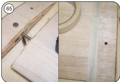
Öffnung für Magnet M 13 von aussen mit Klebestreifen verschliessen, Fläche mit M 15 aufstecken, mit Kreppband fixieren
