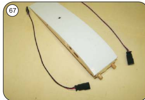
Servoverlängerkabel ( 20 cm ) einbauen
