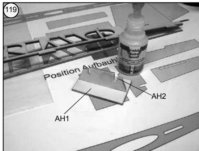
Bild 119 - Die Aufbauhilfe aus den Teilen AH1 und AH2 rechtwinklig zusammenkleben.
