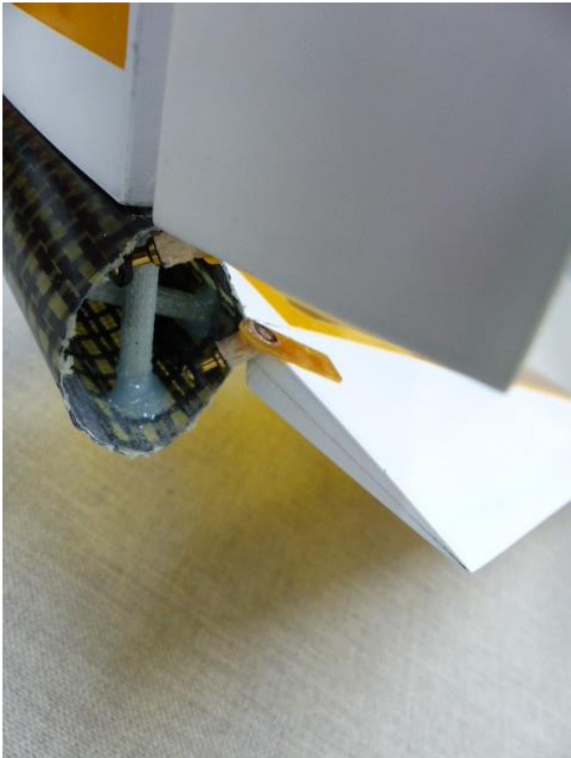
Les tiges de commande en jonc carbone de 3mm commandent en direct les parties mobiles
